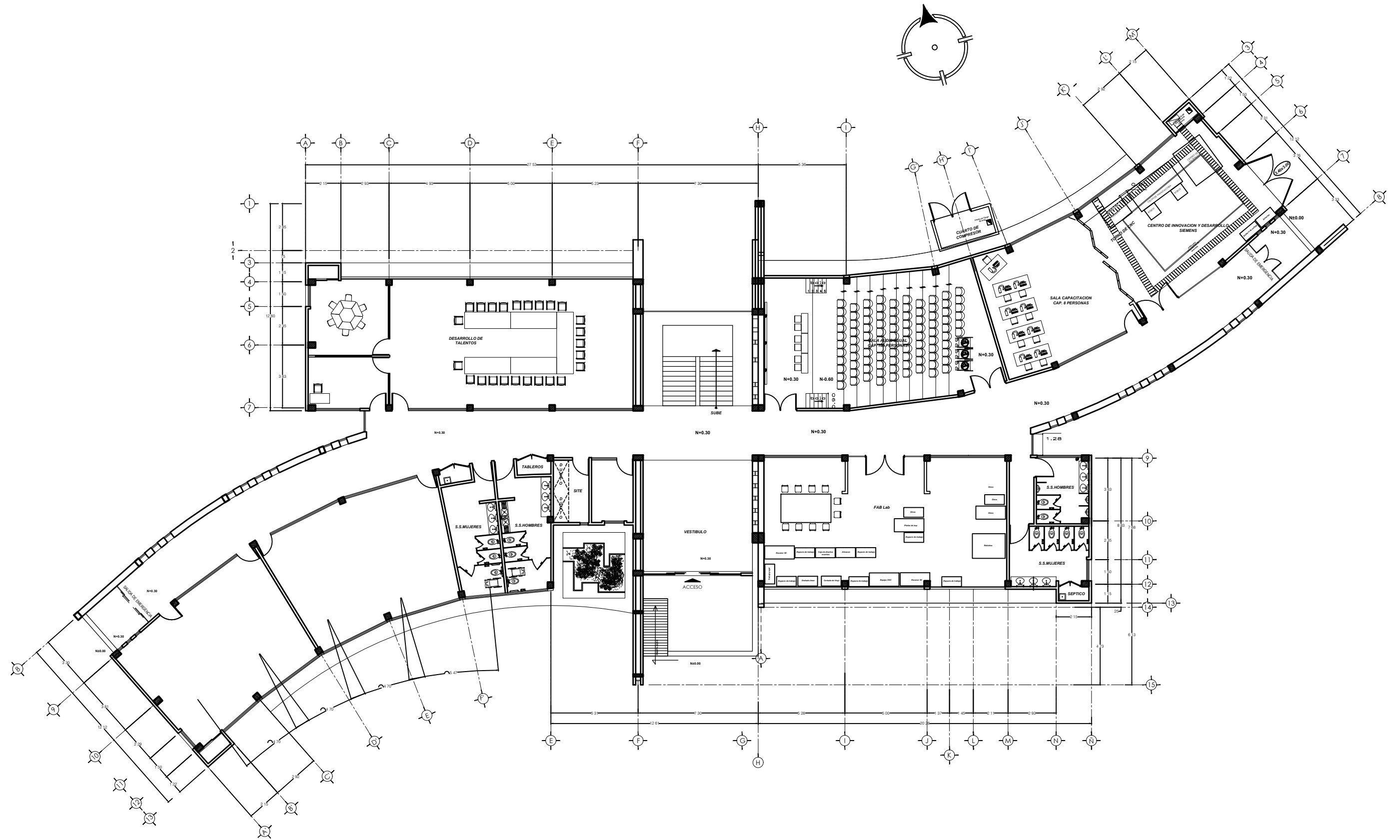
Planta Baja PLANTAS ARQUITECTONICAS CIC 4.0
